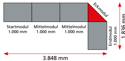
Außenmaße Theken-Set 2*
