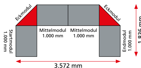
Außenmaße Theken-Set 3*
