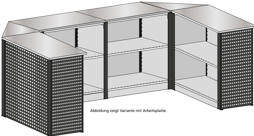
Außenmaße Theken-Set 3*
