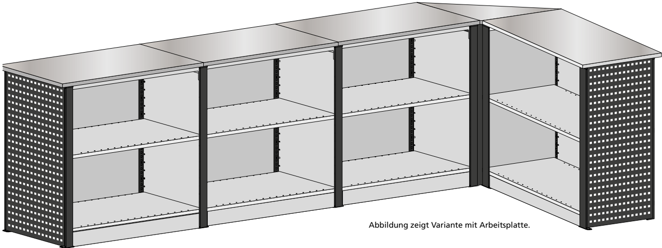
Außenmaße Theken-Set 2*
